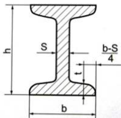
Рисунок 6. Двутавровая балка.
