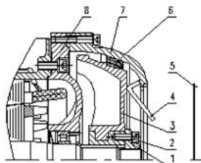
Рисунок 14. Описание регулировки тормозной системы тельфера 10т .
