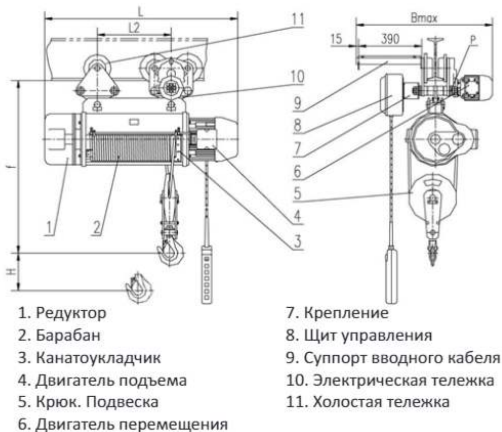
Рисунок 2. Схема тельфера 0,5-5 тонн с тележкой (высота подъема 12 и более метров).
