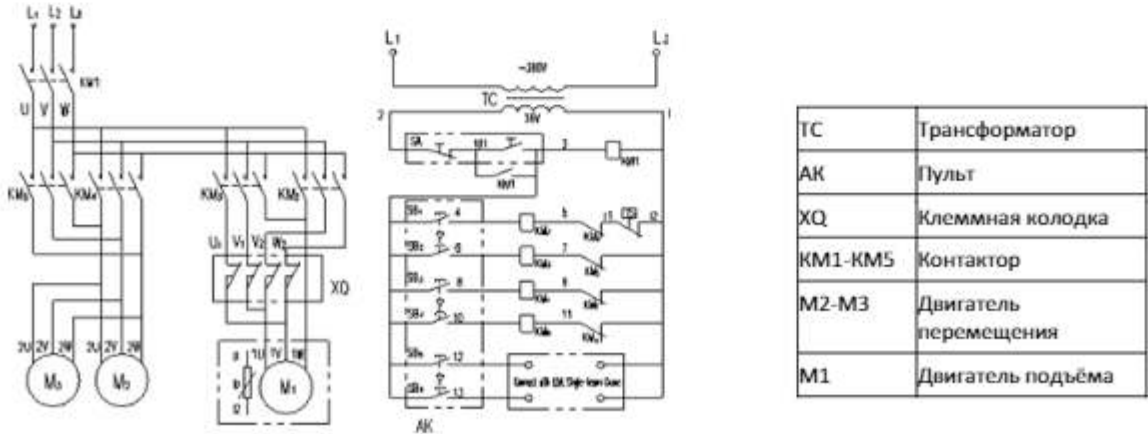
Рисунок 9.Электрическая схема тельфера.
