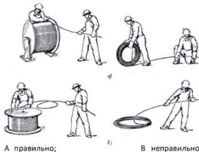
Рисунок 12. Разматывание каната.
