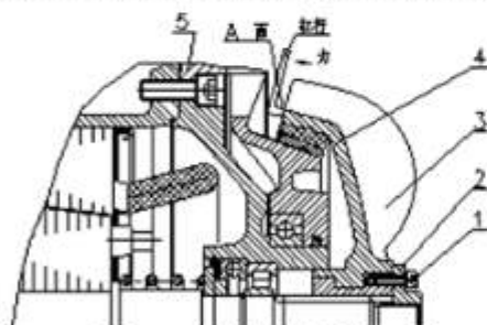
Рисунок 13. Описание регулировки тормозной системы тельферов 0,5 -5т.
