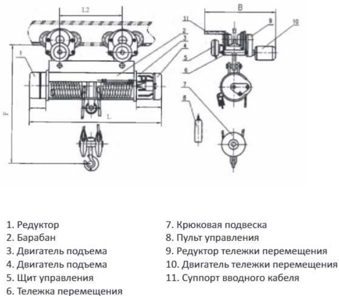
Рисунок 3. Схема тельфера 10 тонн
