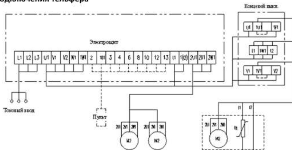
Рисунок 10. Схема подключения тельфера
